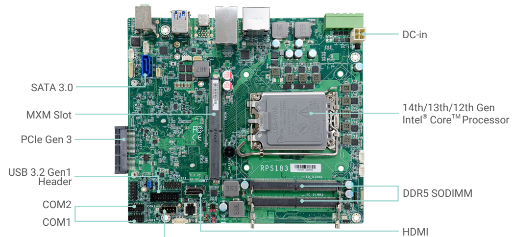
Top View (RPS183-H610E)
